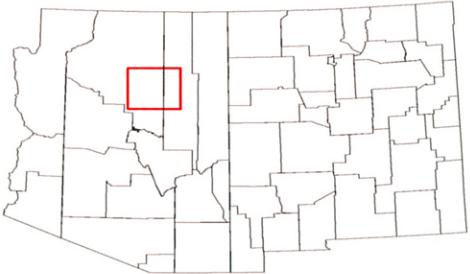
Context Map
